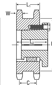
TIPO B BUCHA MST®
