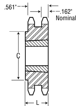
Bucha Taper Tipo B
