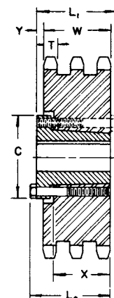
Tipo B Bucha QD
