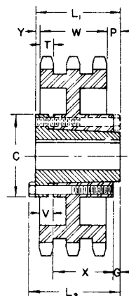
Tipo C 3 Bucha QD
