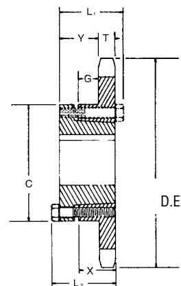
Tipo B Bucha QD
