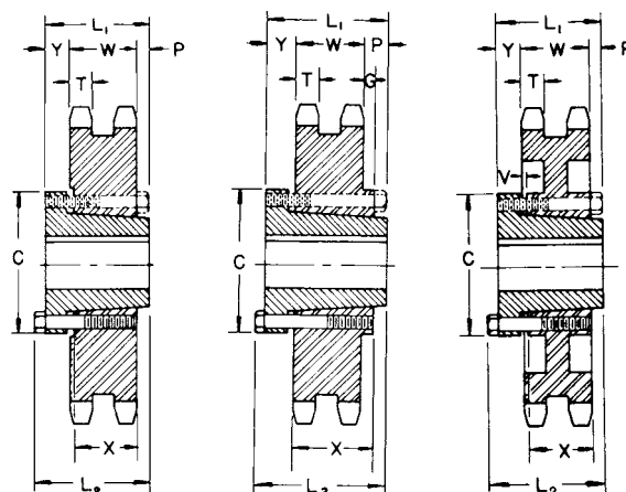
Bucha QD Tipo C 1
