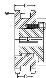
Tipo B Bucha MST
