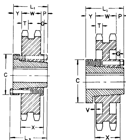
Bucha QD Tipo C 2
