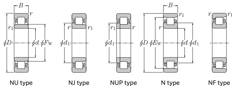
d 170 ~ 220mm
