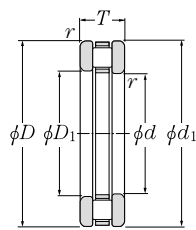
811 type (Bearing)
